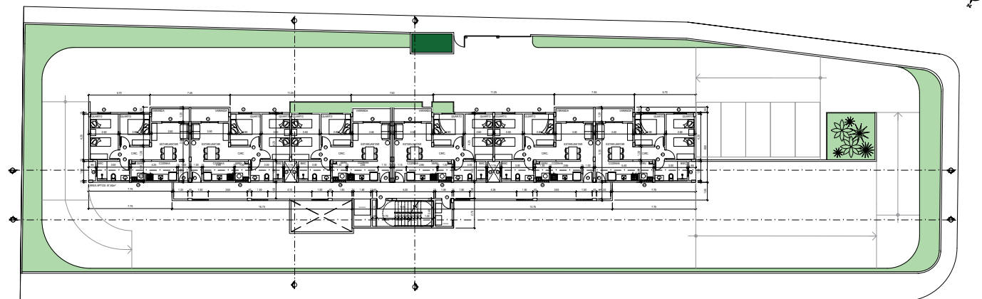
04 PLANTA BAIXA PAVIMENTO TIPO SENHA 1108
