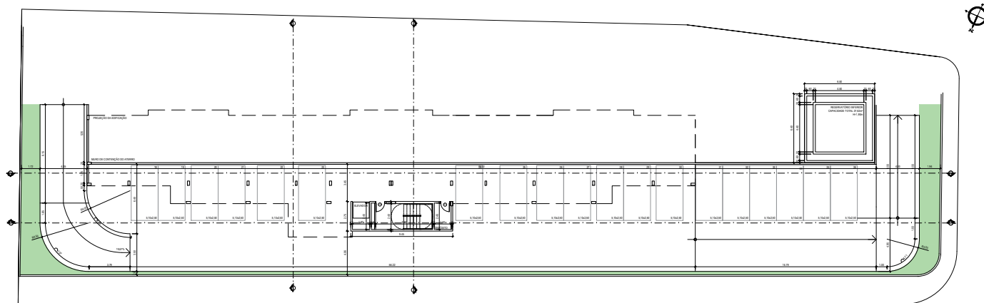
03 PLANTA BAIXA SUBSOLO SENHA 1108
