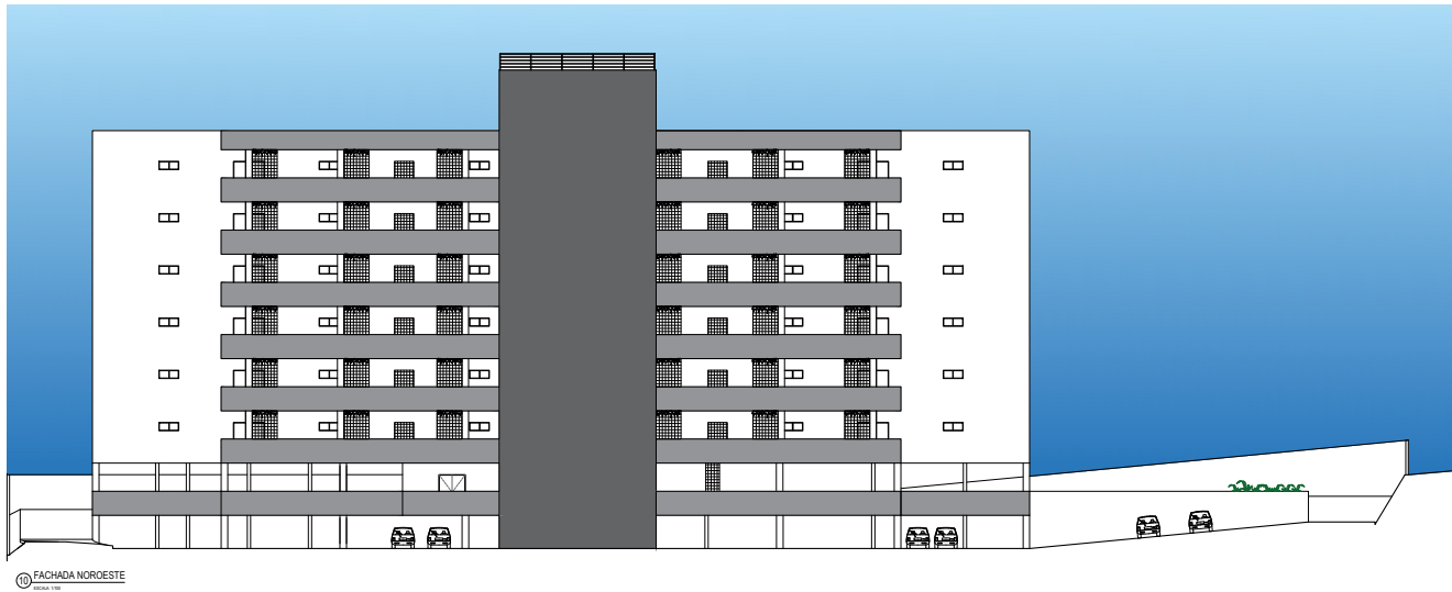
FACHADA NOROESTE
