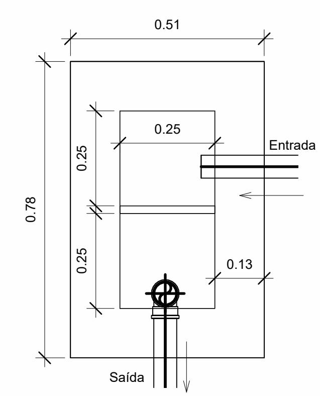
8 Caixa de Gordura 1 : 10
