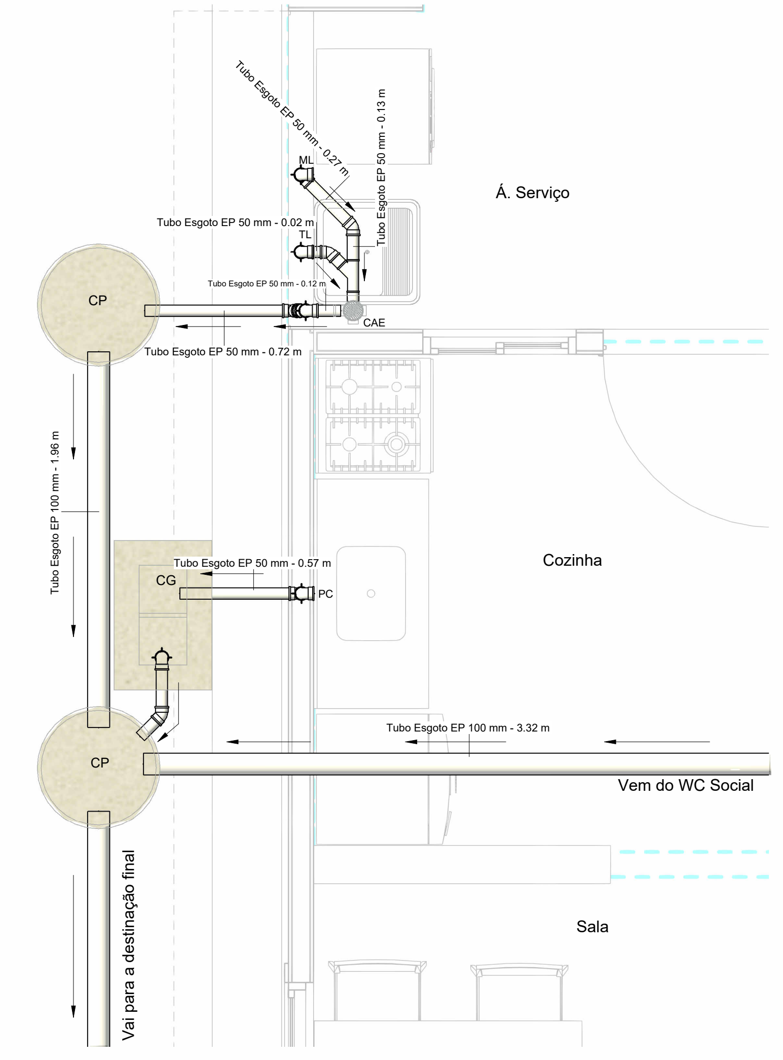
4 Sanit PB Cozinha/Á. Serviço 1 : 20
