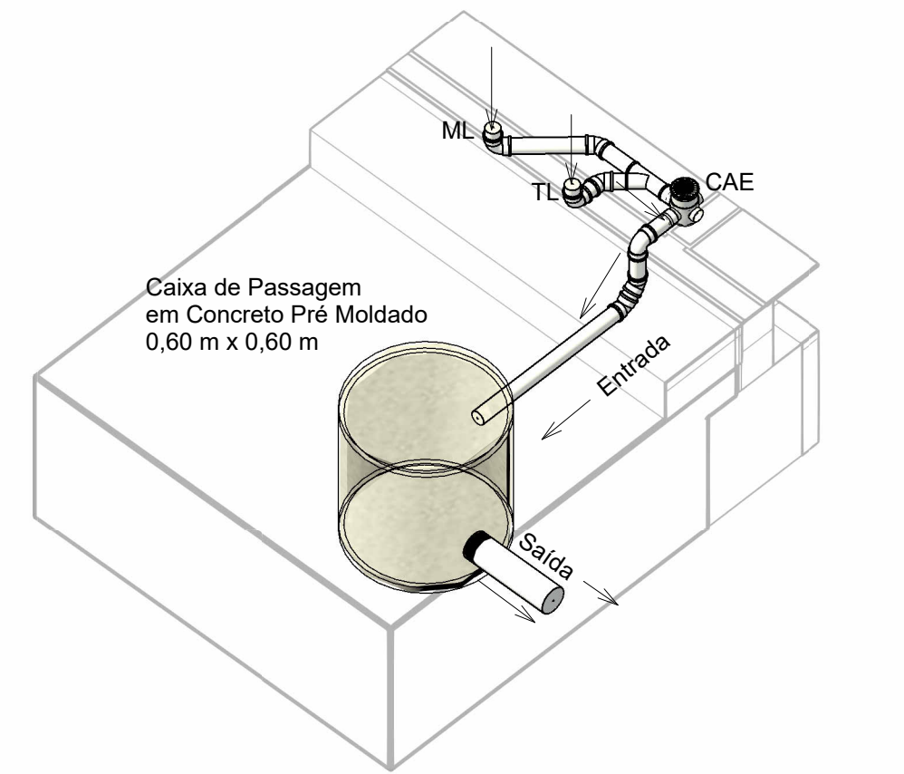
7 Caixa de Passagem
