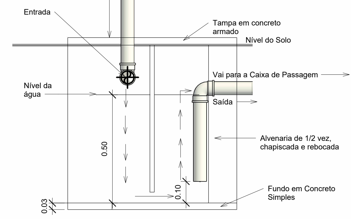
5 Det da Caixa de Gordura 1 : 10
