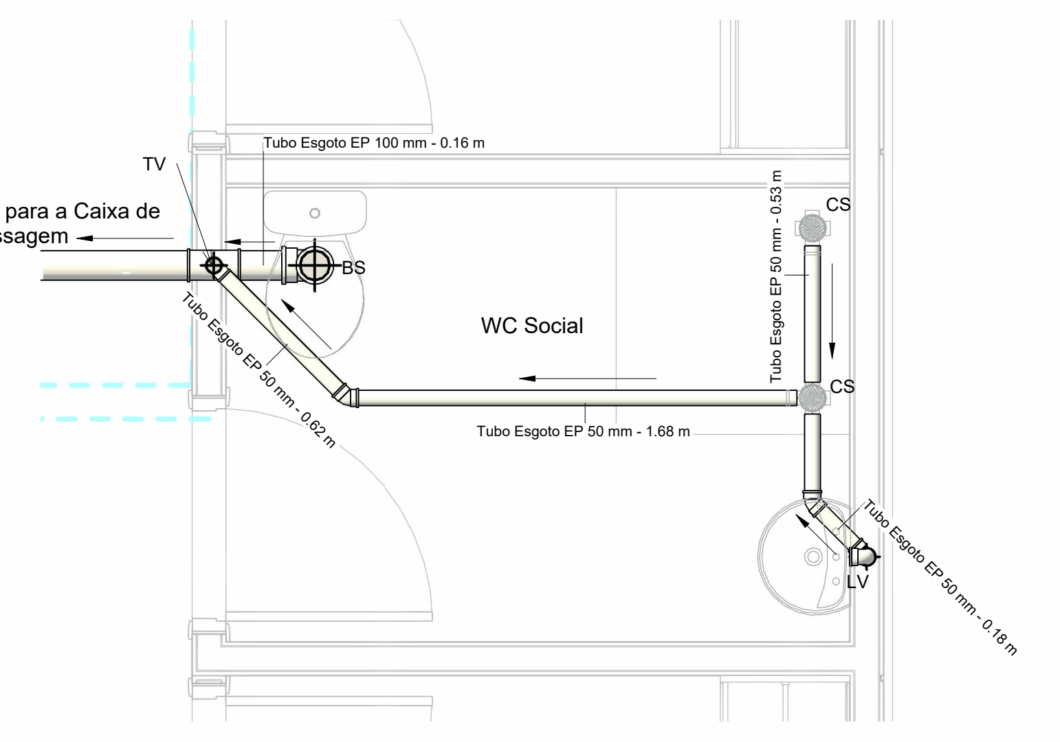
3 Sanitário Planta Baixa WC 1 : 20
