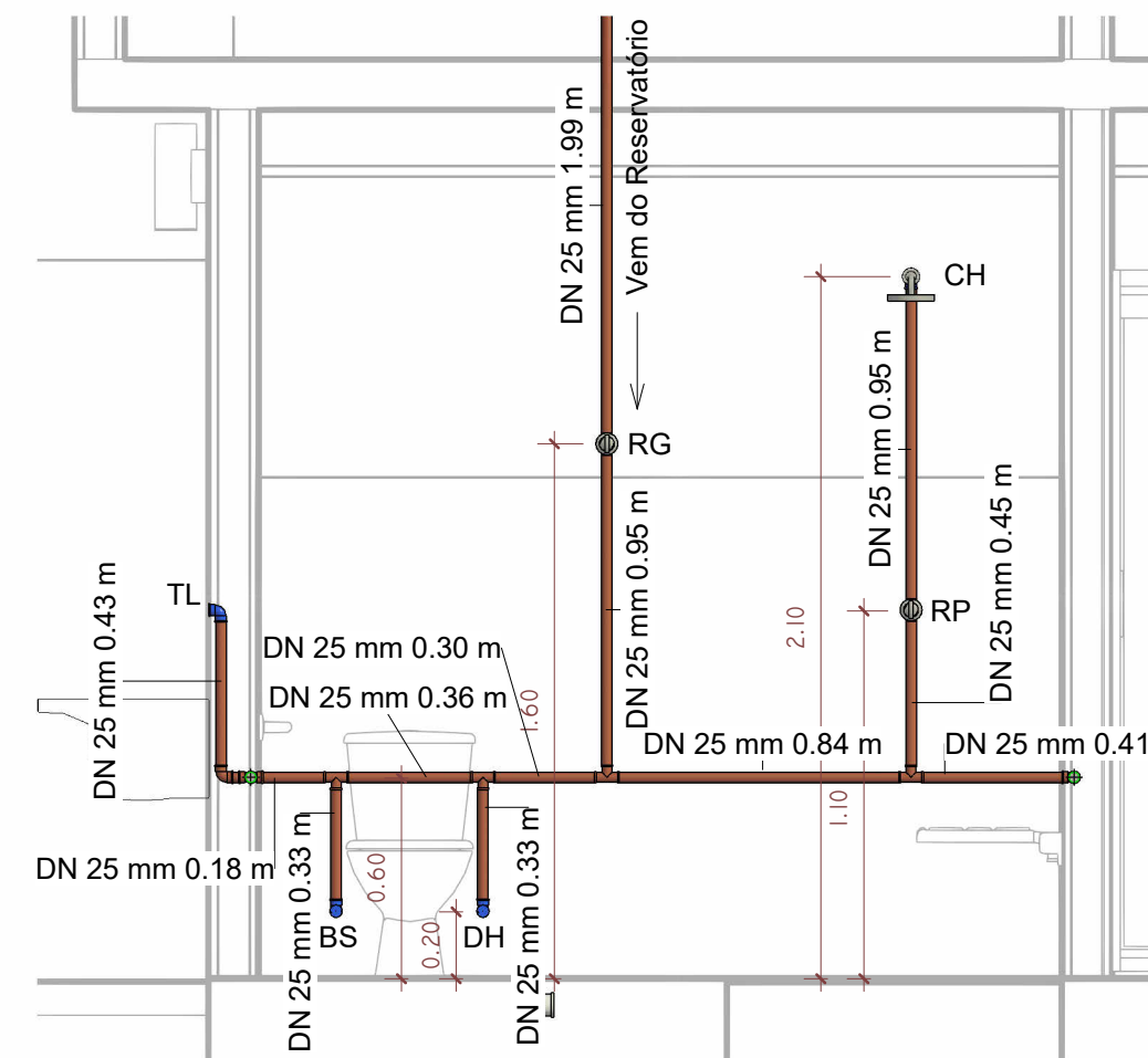
6 Elevação WC - Casas 02 e 04 1 : 25
