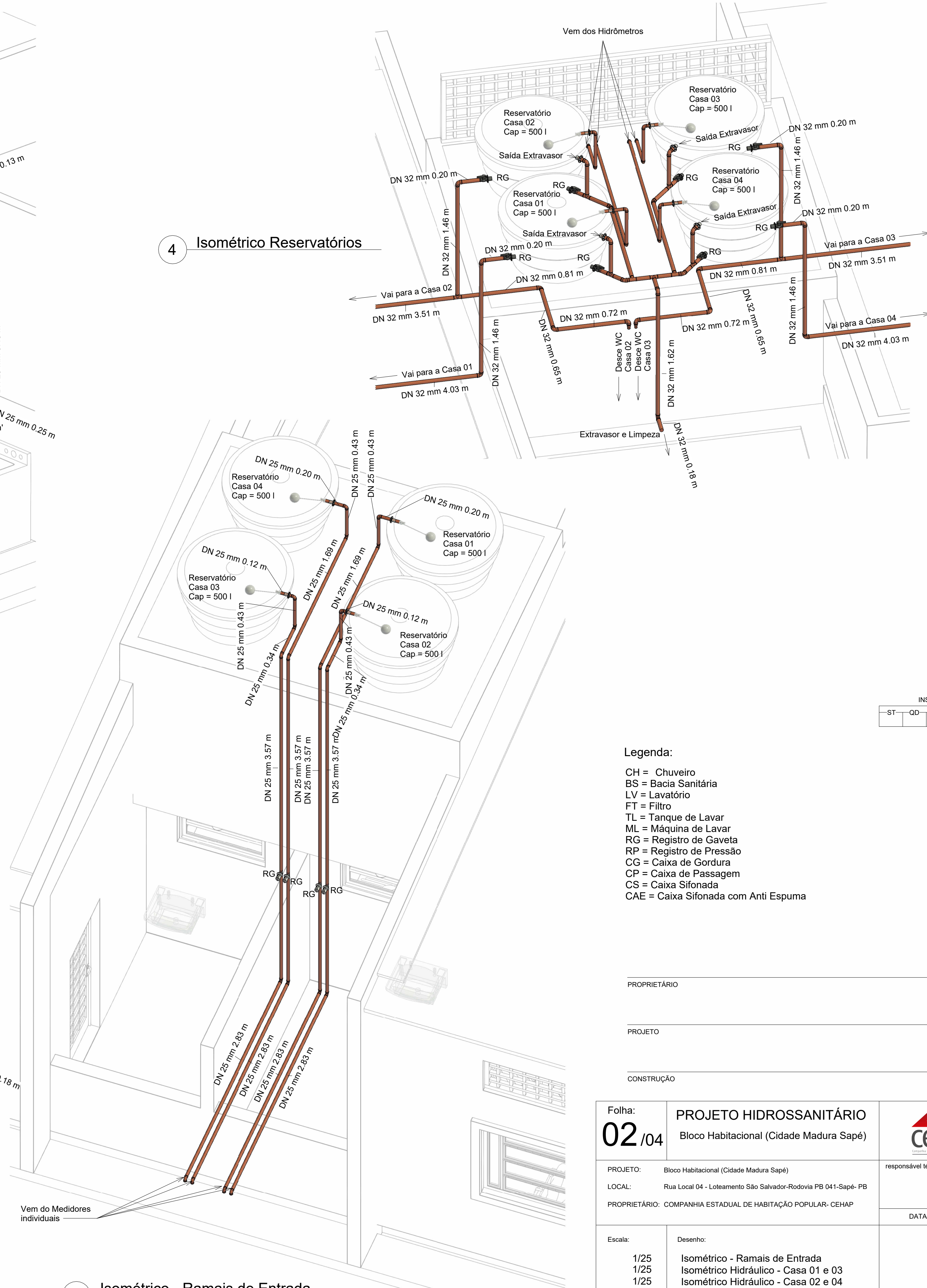
1 Isométrico - Ramais de Entrada
