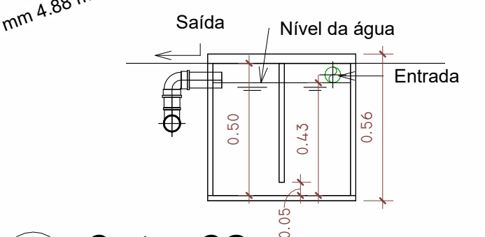
6 Corte - CG
