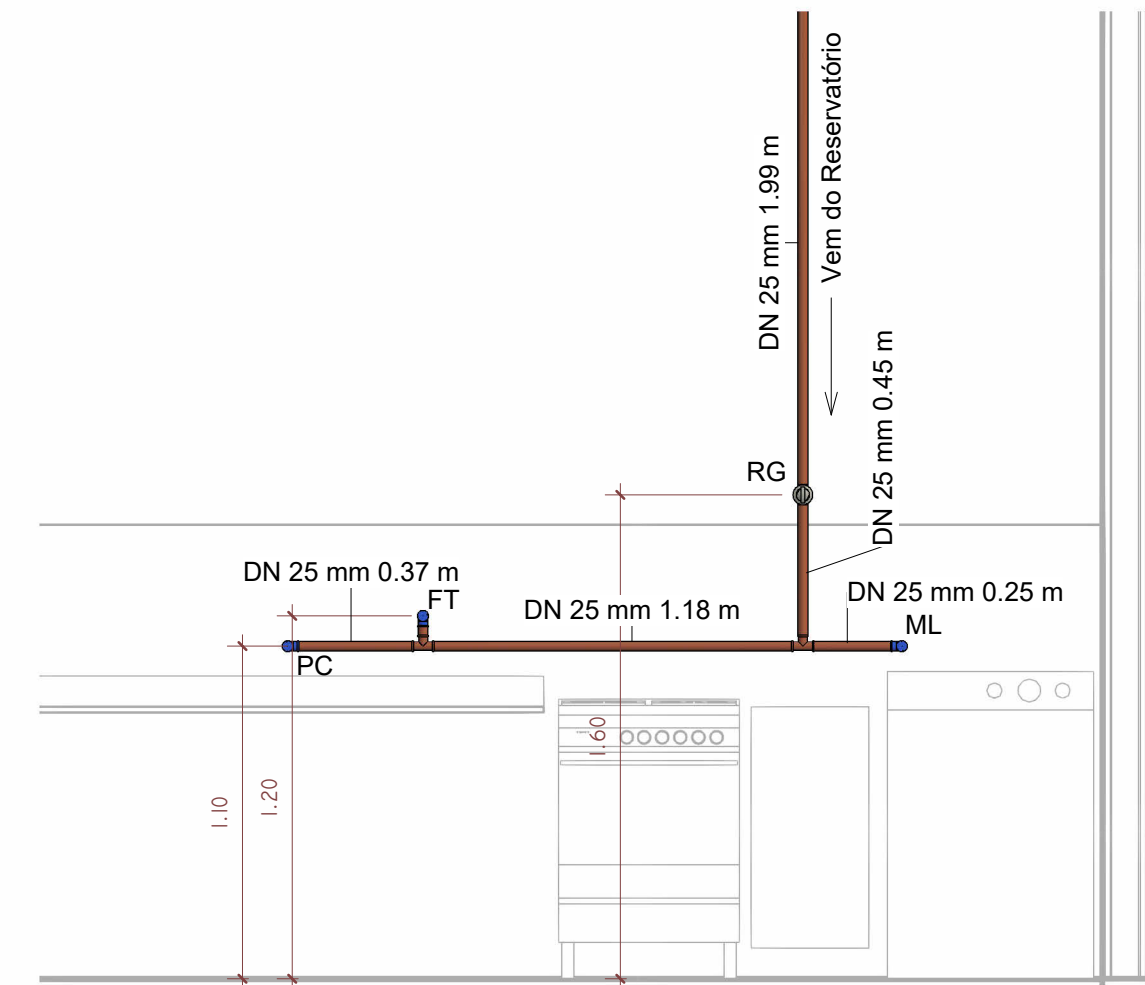
4 Elevação Cozinha - Casas 02 e 04 1 : 25
