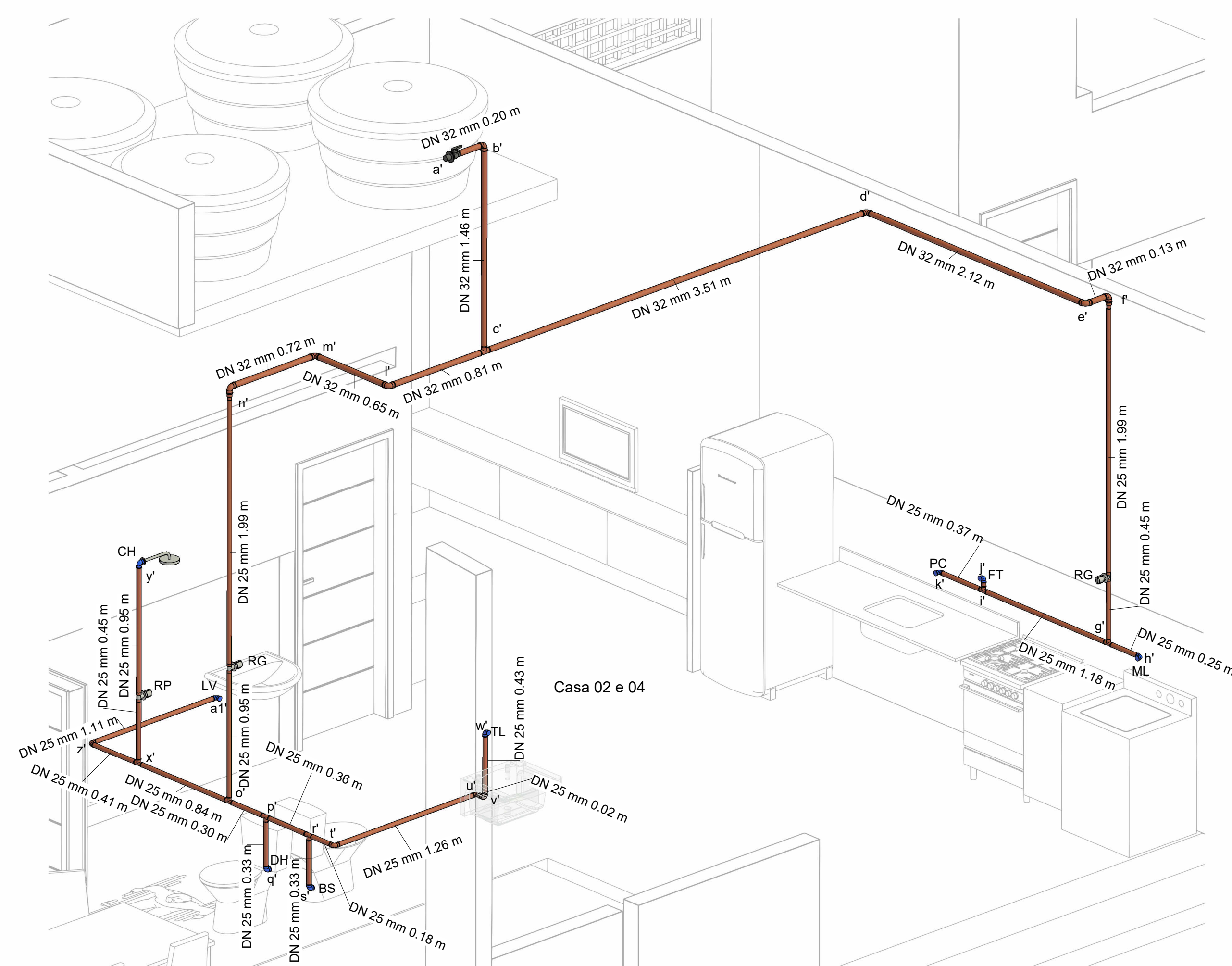
3 Isométrico Hidráulico - Casa 02 e 04
