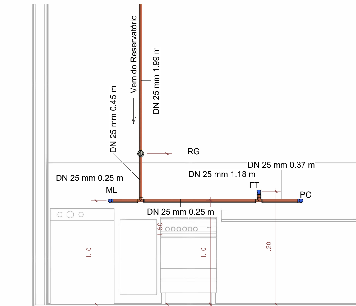
3 Elevação Cozinha - Casas 01 e 03 1 : 25
