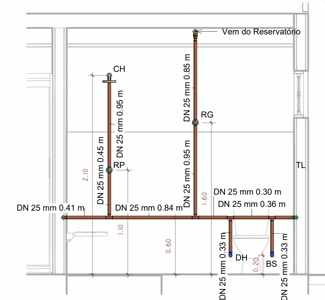
5 Elevação WC - Casas 01 e 03 1 : 25
