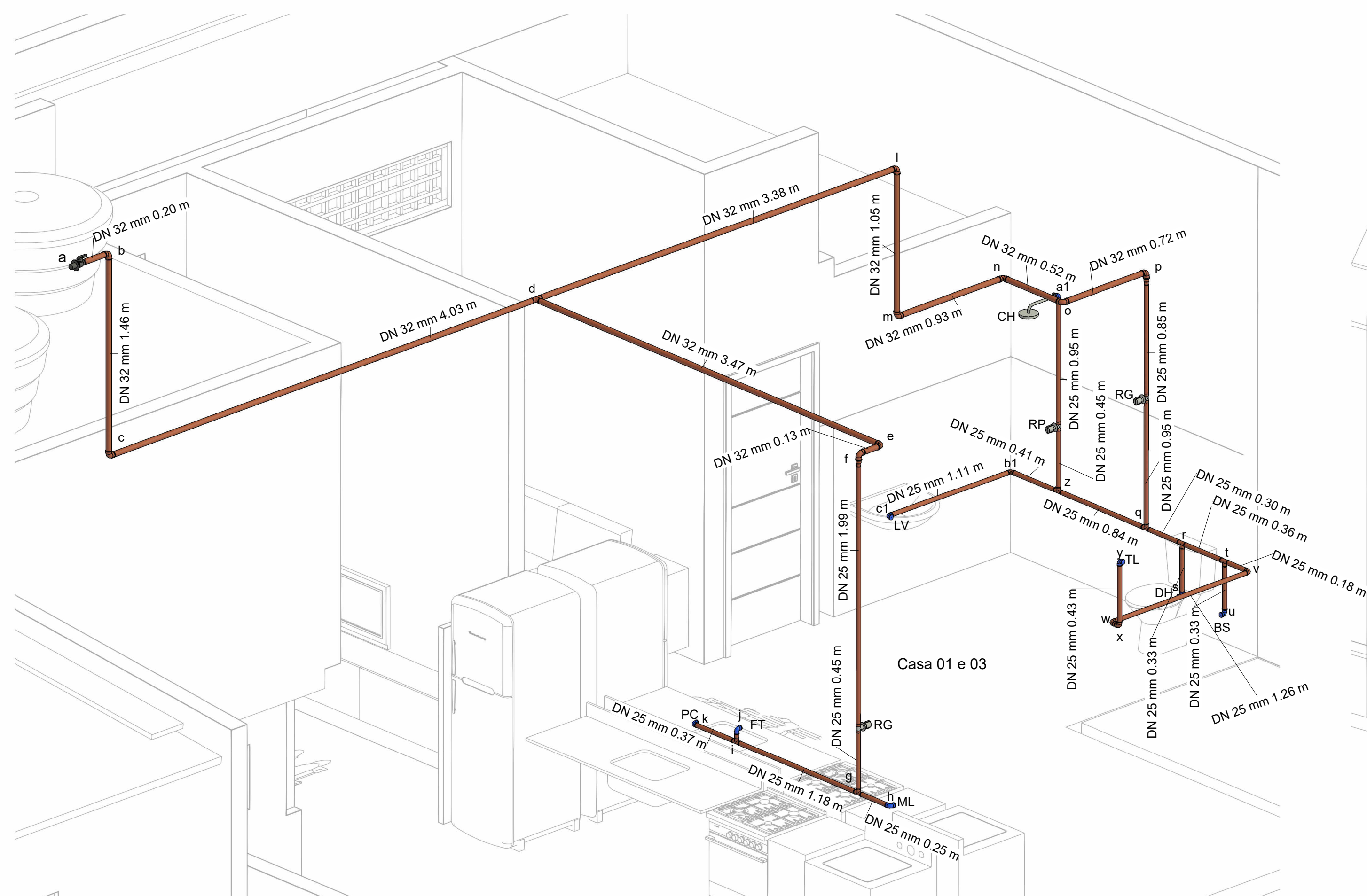
2 Isométrico Hidráulico - Casa 01 e 03
