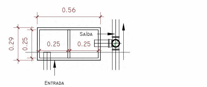
5 Planta - CG
