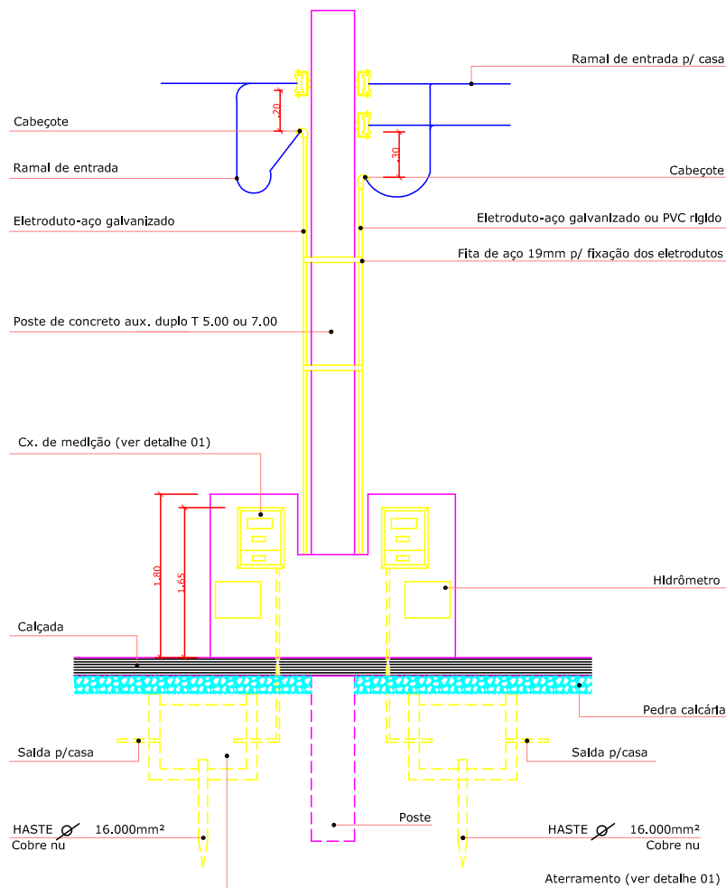
DETALHE DE INSTALAÇÃO-MEDIÇÃO EM MURETA ESCALA 1/75
