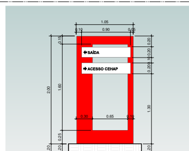
9 VISTA FRONTAL PLACA 07 1:20
