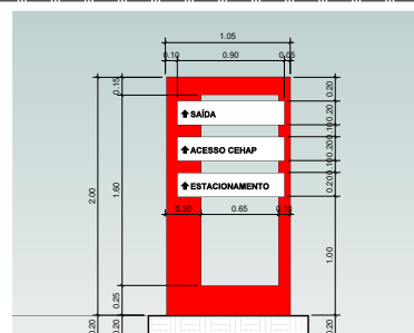
8 VISTA FRONTAL PLACA 06 1:20
