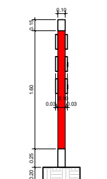
4 CORTE PLACA 05 1:20
