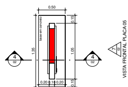
1 PLACA 05- Planta Baixa- sinalização 1:20
