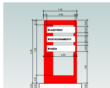
7 VISTA FRONTAL PLACA 05 1:20
