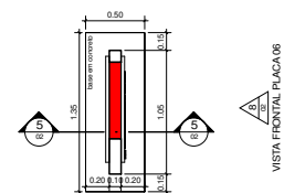
2 PLACA 06- Planta Baixa- sinalização 1:20
